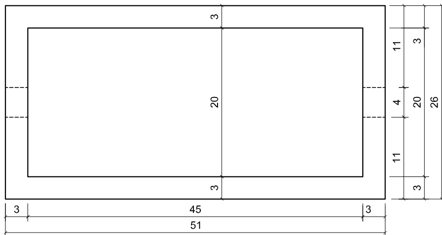
01 Planta Baixa Escala 1:5
